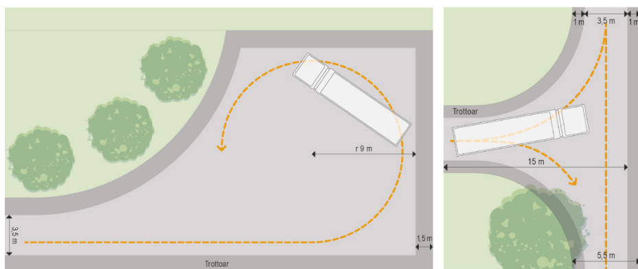
Alternativ på vändplatser för baklastande tömningsfordon. Bild: Sara Sundin, Ramboll.
