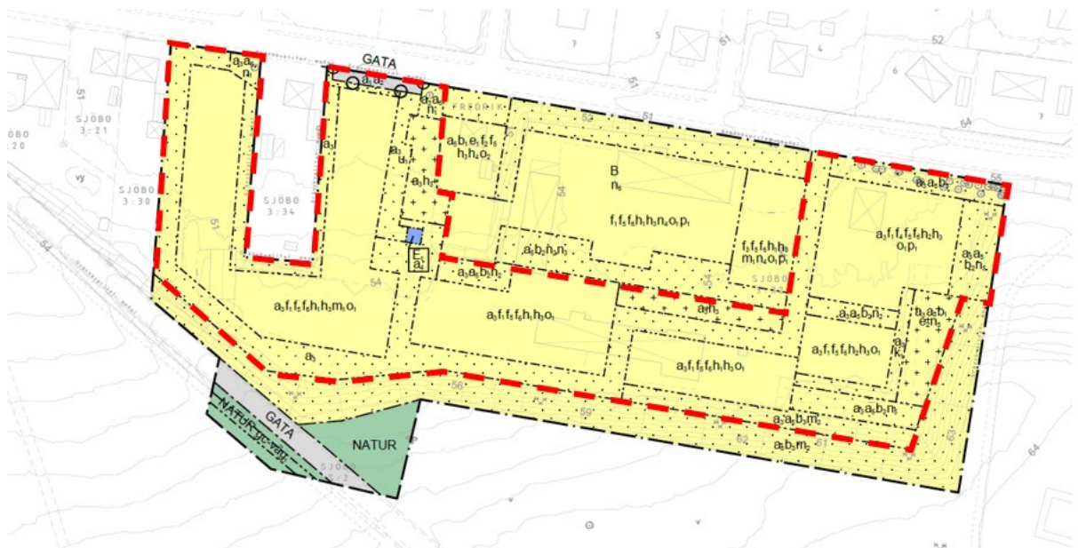
Utsnitt av plankartan där röd streckad linje visar avgränsningen för vilken del av planområdet som omfattas av villkor om startbesked kopplat till markföroreningar, planbestämmelserna a1, a2, a3 och a4.
