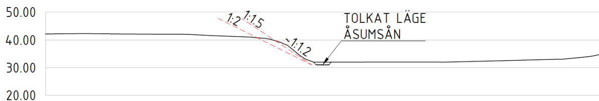
Figur 3.5.3-2 Bedömd utbredning av ras för principsektion B, centrala Sjöbo.
