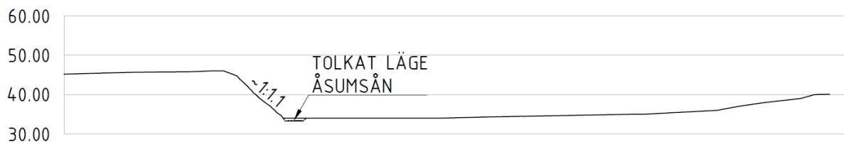
Figur 3.5.1-2 Principsektion A för centrala Sjöbo.
