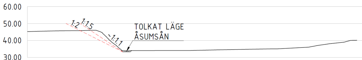
Figur 3.5.3-1 Bedömd utbredning av ras för principsektion A, centrala Sjöbo.
