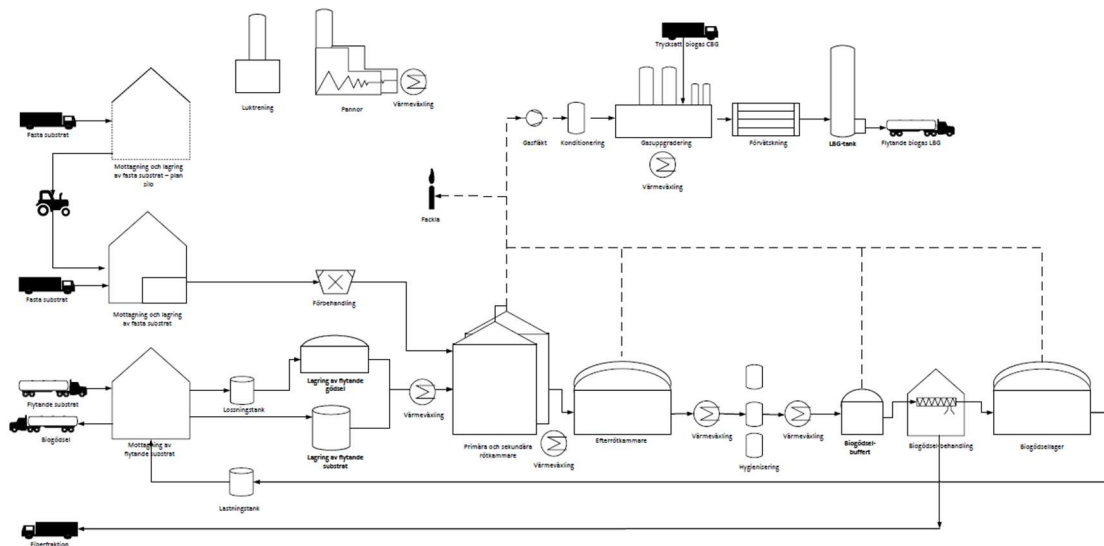
Figur 7. Processbild av verksamheten.
