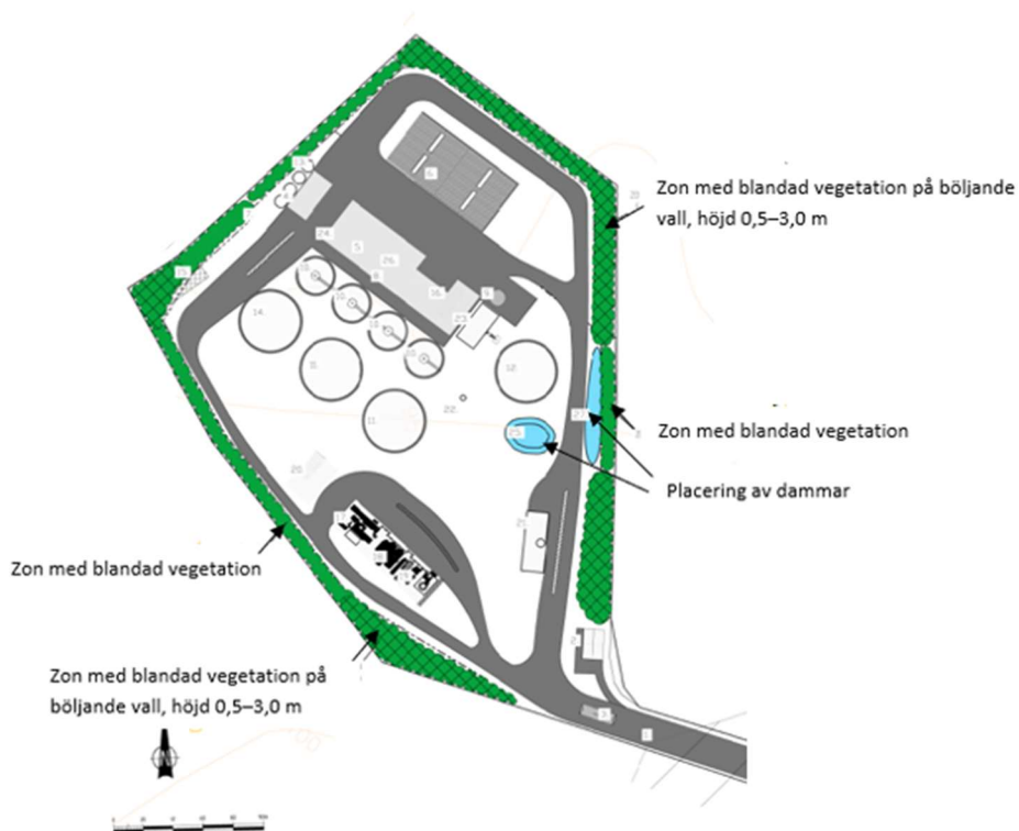
Figur 20. Figuren visar placering av dammar.
