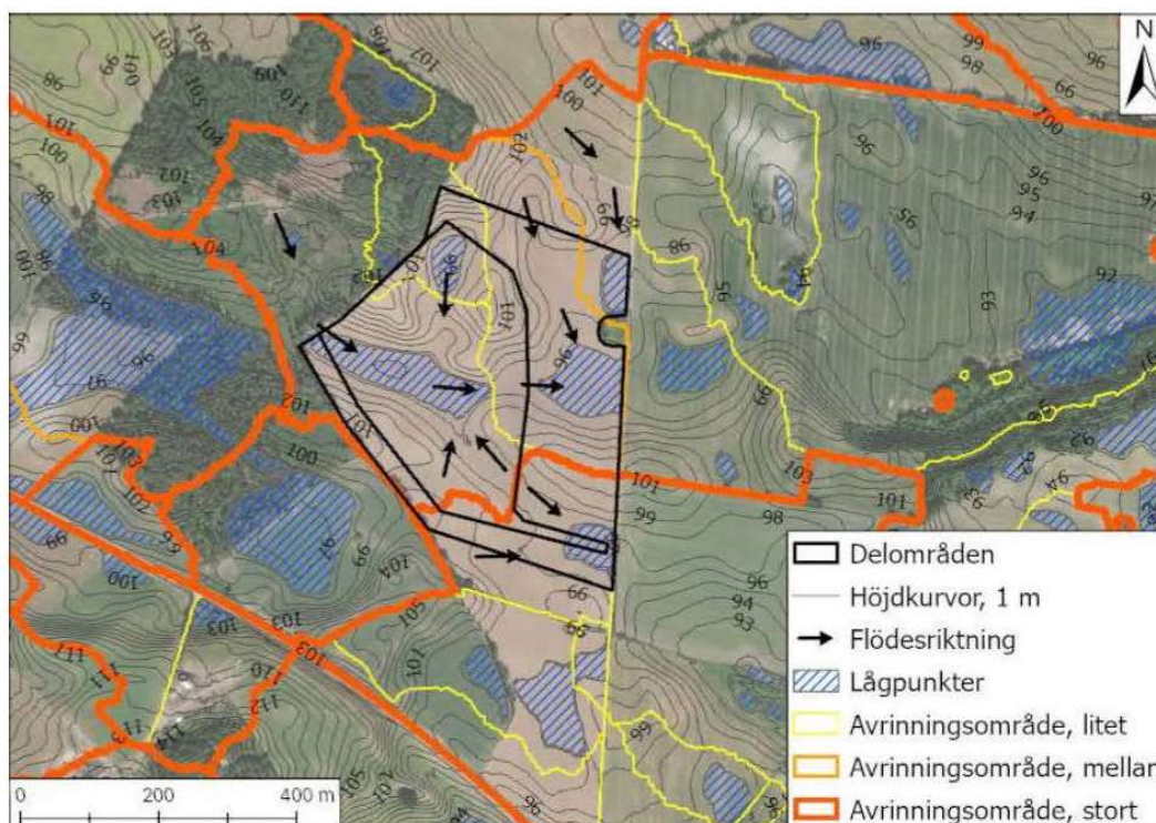
Figur 19. Höjder, avrinningsområde, flödesriktningar och lågpunkter inom området. (Källa: Dagvattenutredning, WSP 2023)
