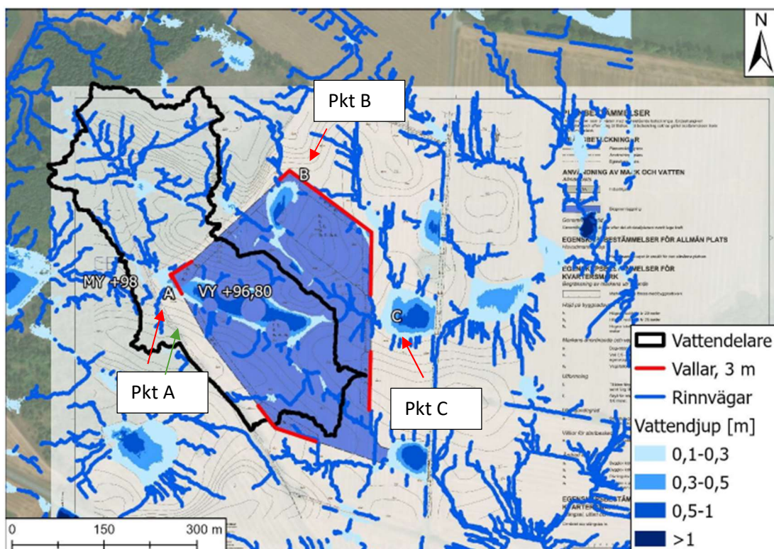
Figur 21. Rinnvägar och vattendelare med planerade vallar. Källa. Dagvattenutredning WSP 2024-01-22.
